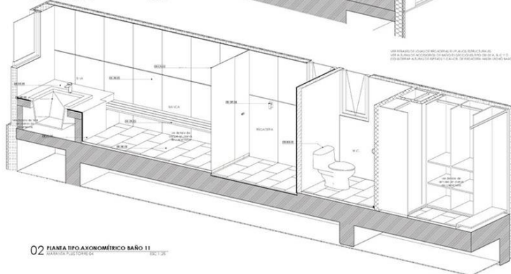
01 PLANTA TIPO AXONOMÉTRICO BAÑO 11 MARANTA PLUS TORRE 04
