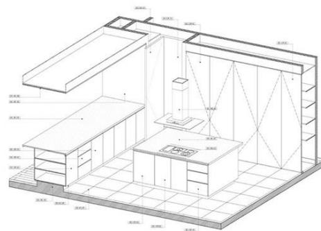
03 PLANTA JARDÍN, VISTA AXONOMÉTRICA COCINA 01 MARANTA PLUS TORRE 04
